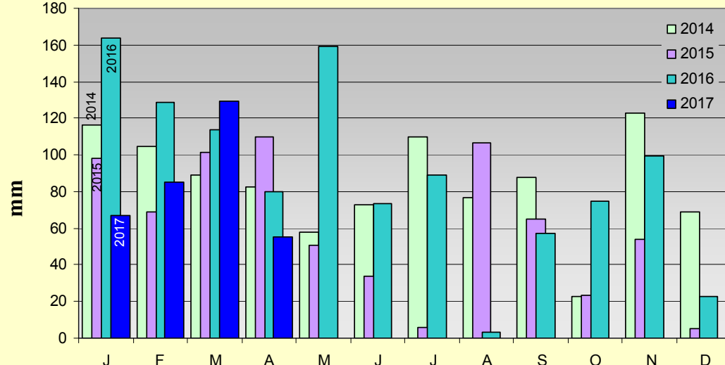
Pluviométrie totale mensuelle
