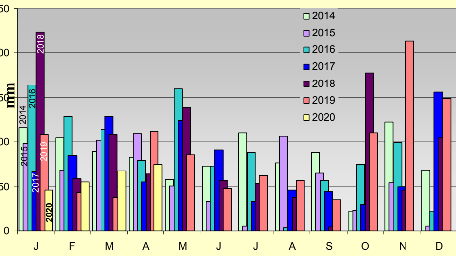
Pluviométrie totale mensuelle
