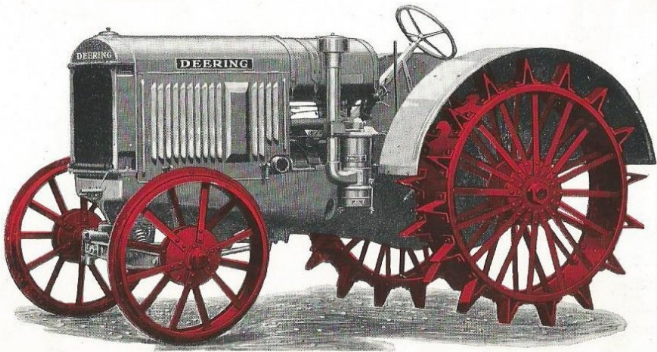
Tracteur " DEERING " 22-36 (Noter le filtre à air).
