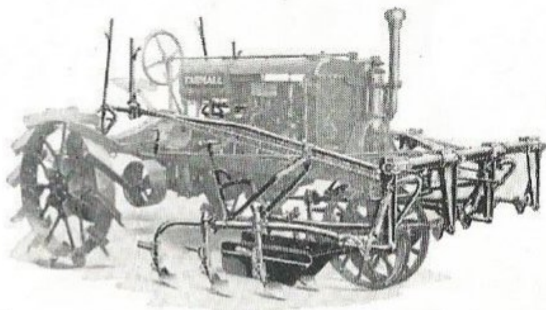
Cultivateur "porté".
