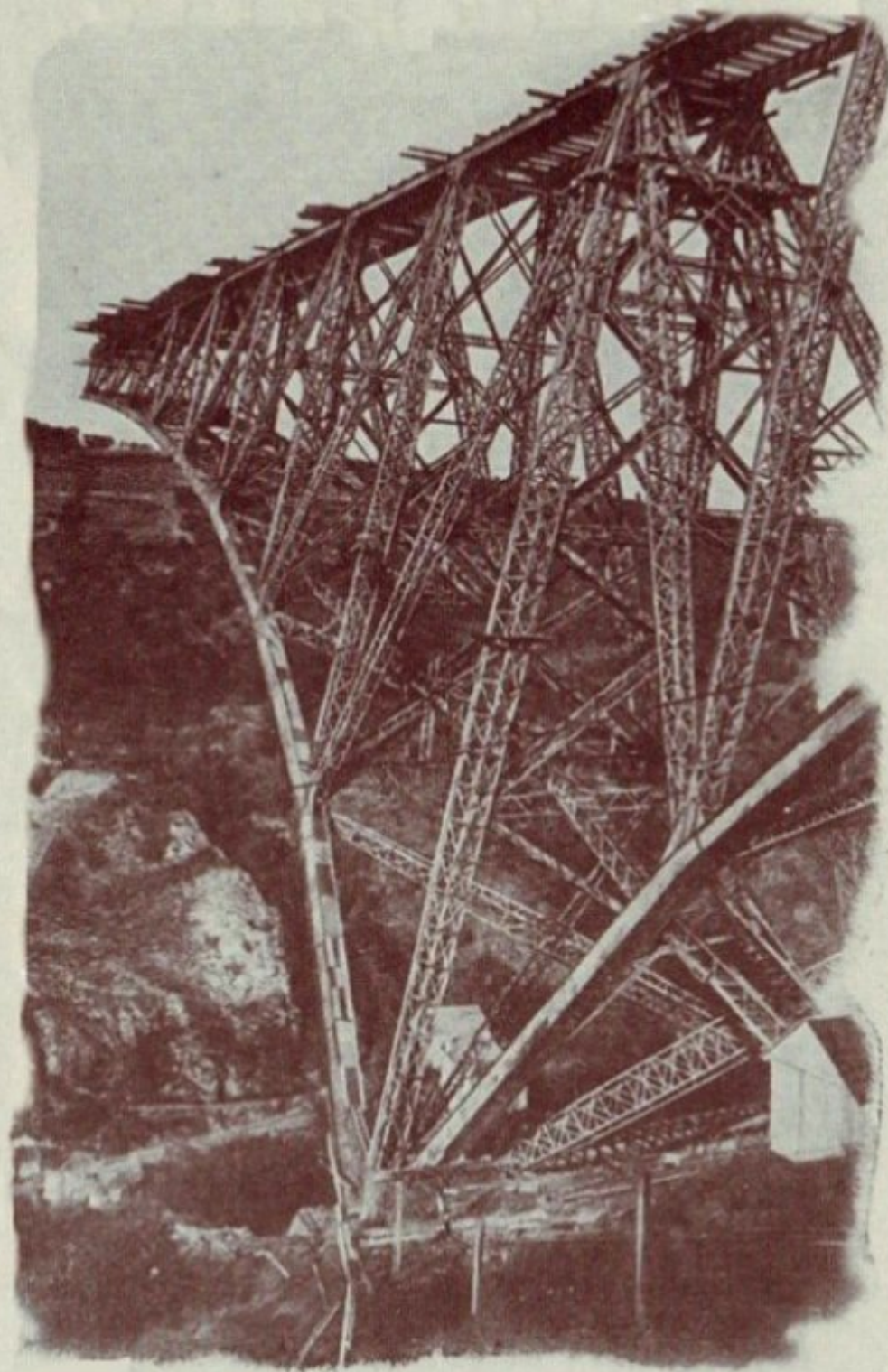
Le Viaduc du Viaur en construction (Tarn - Aveyron)
